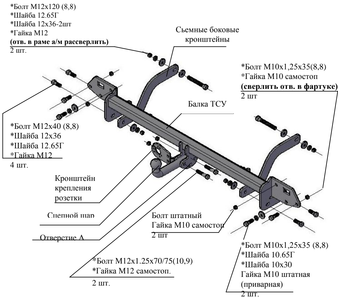
Рис.1 Тягово-сцепное устройство ТСУ 9620
