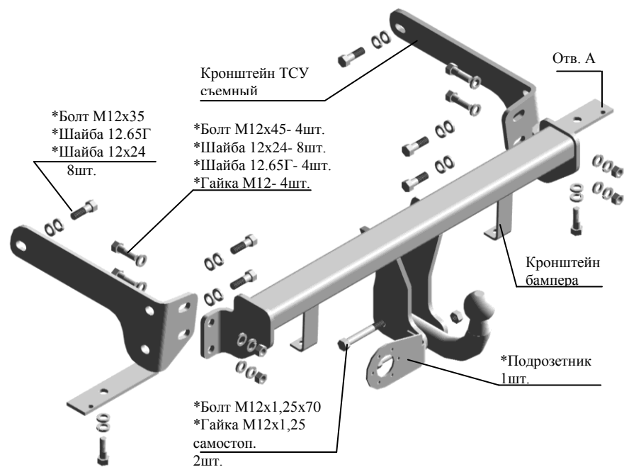
Рис.1 Тягово-сцепное устройство 9430
