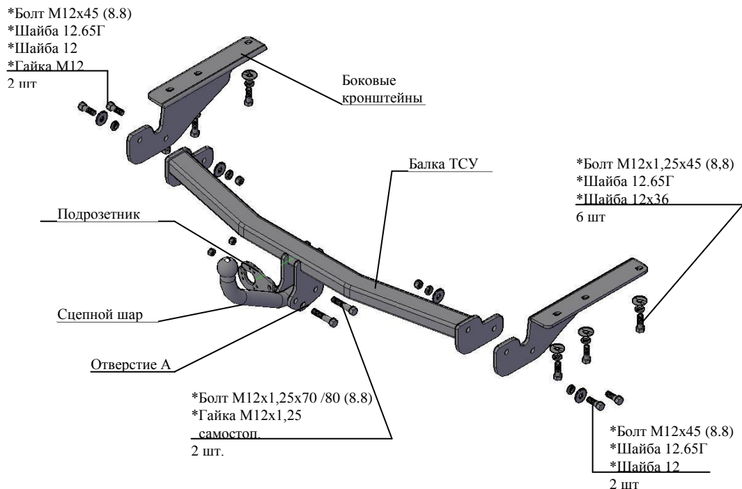
Рис.1 Тягово-сцепное устройство 7830.
