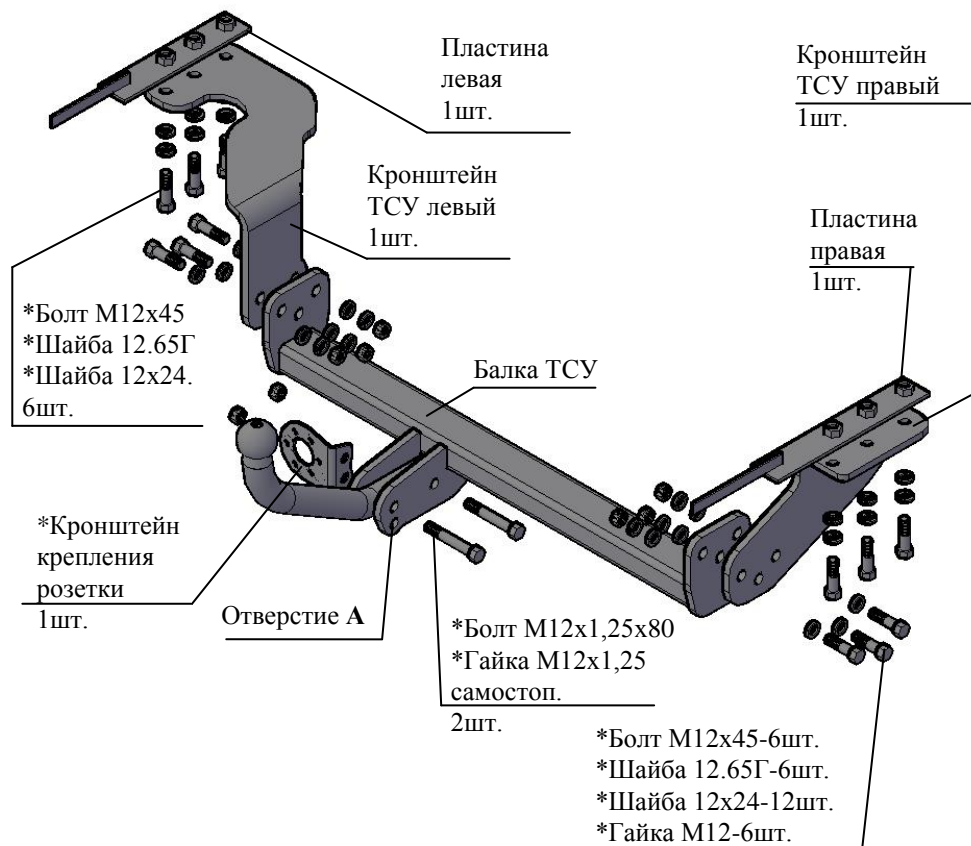
Рис.1 Тягово-цепное устройство 7710
